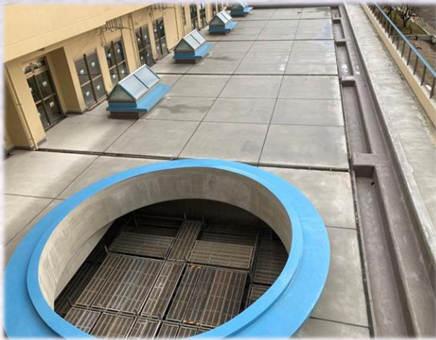
2F テラスガーデン ベンチ部ウレタン防
