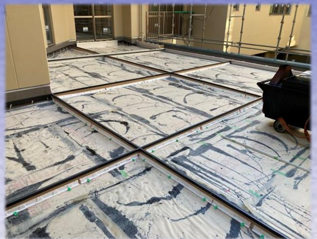
2F 中庭アスファルト防水完了、伸縮目地張り状況
